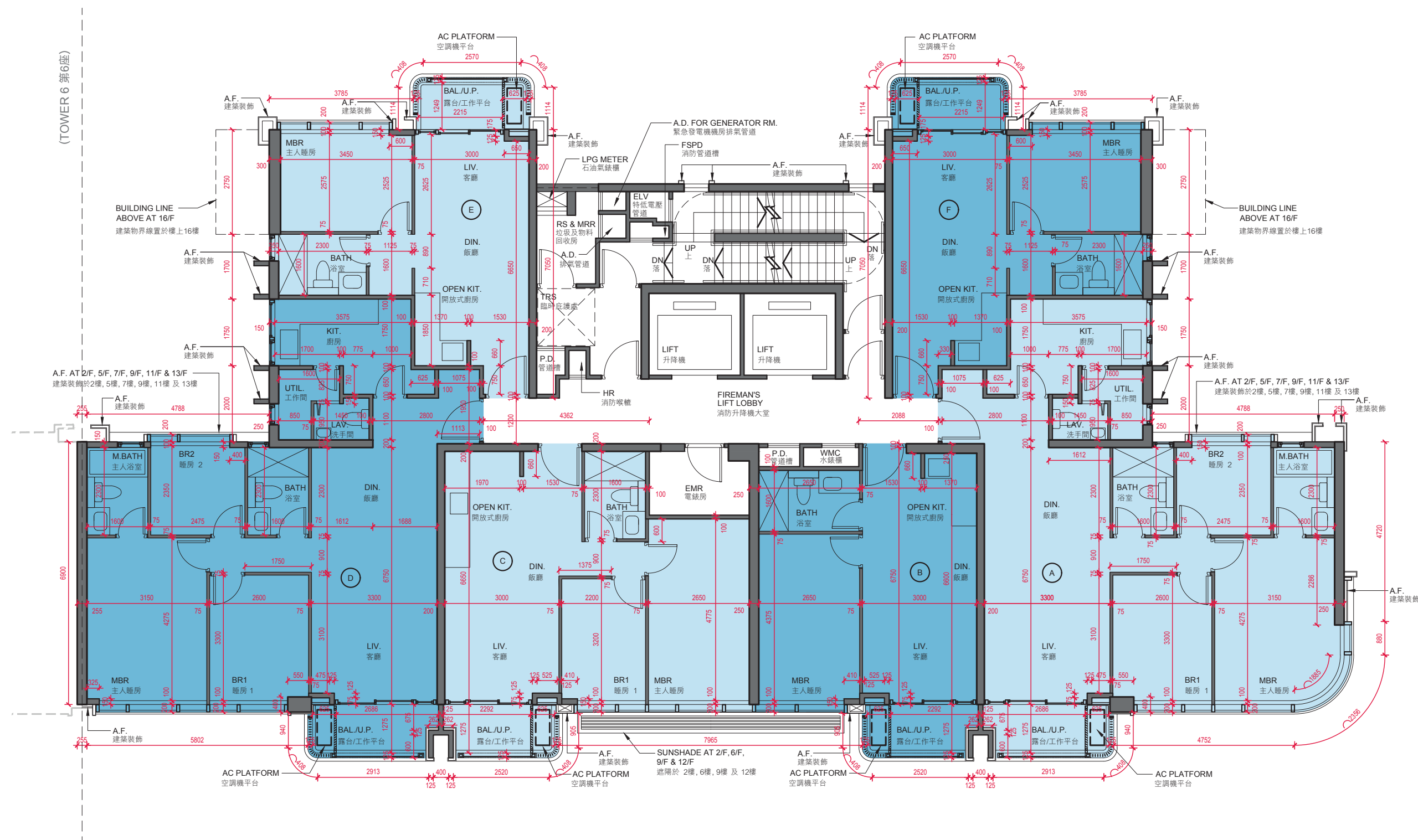
TOWER 3 2/F-3/F, 5/F-13/F, 15/F FLOOR PLAN 第3座 2樓至3樓，5樓至13樓，15樓樓面平面圖
